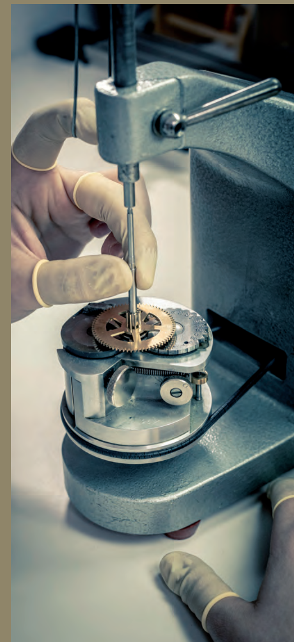
Mit dem Zapfenrolliergerät werden die Räderzapfen auf Hochglanz druckpoliert.
