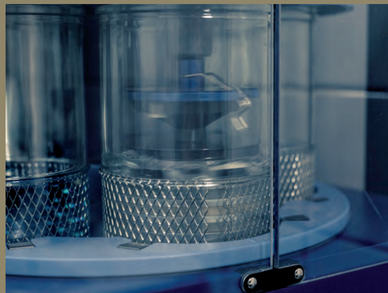
Die Reinigungsmaschine in Aktion. Vollkommene Fettfreiheit und Sauberkeit sind das Ziel, das es zu erreichen gilt.
